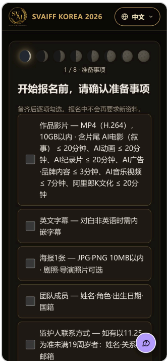
手机画面（390×844）
