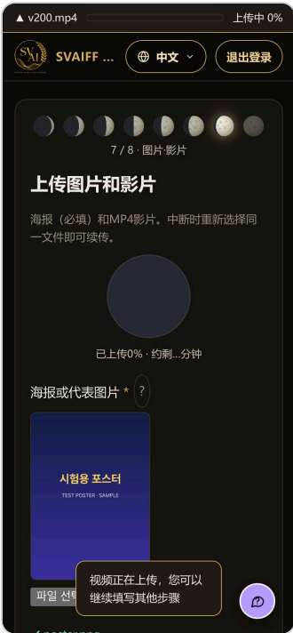
手机画面（390×844）
